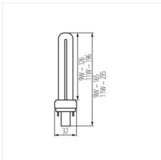
T1U-9W/K
