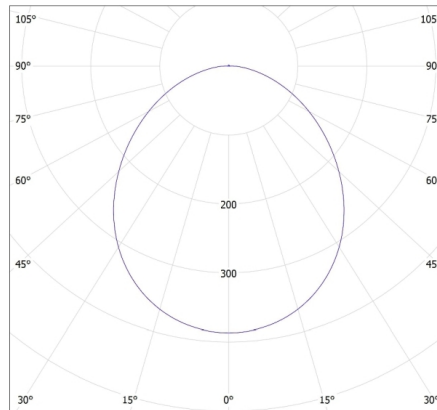
KANLUX S.A. (akt 22821) TOMI LED7W GU10-WW / Krzywa rozsyłu światła (biegunowo)
