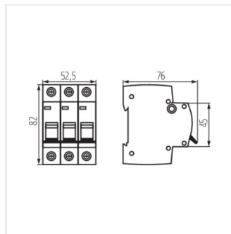
KMB6-B20/3
