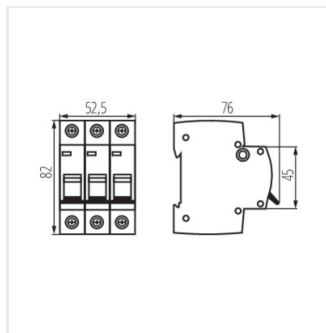
KMB6-B25/3
