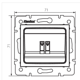
DOMO 01-1450-002 bi
