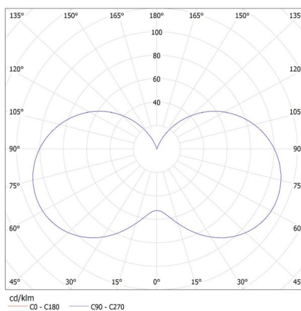
KANLUX S.A. (kat 27296) IQ-LED C37E14 5,5W-CW / LDC (Polar)
