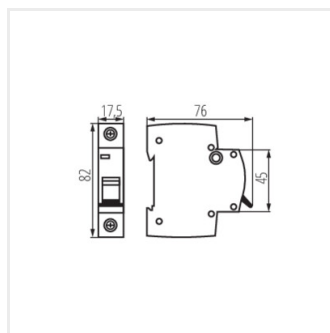
KMB10-C32/1
