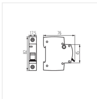
KMB10-C40/1
