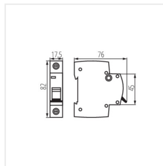
KMB10-C25/1
