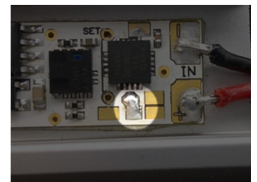
Obr.3 - Propojka J1
