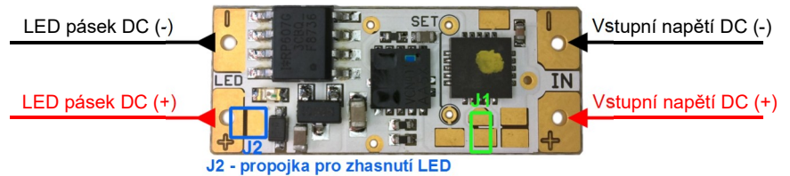
Obr. 1 - Zapojení vývodů modulu
